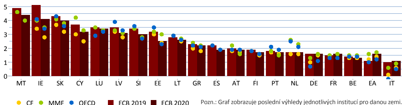
Výhledy růstu HDP v zemích eurozóny pro rok 2019 a 2020, %
