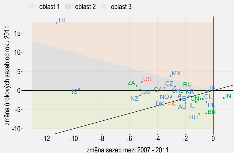
Graf 4 – Změny základních úrokových sazeb centrálních bank
