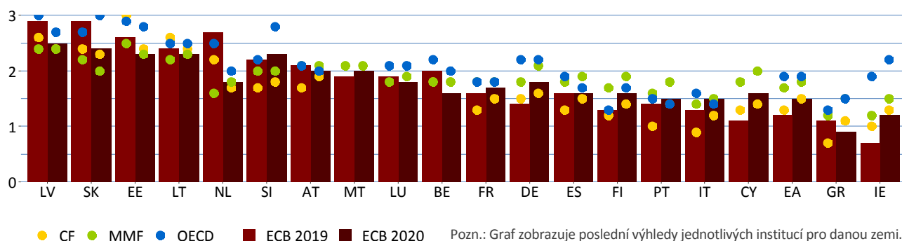
Výhledy inflace v zemích eurozóny pro rok 2019 a 2020, %
