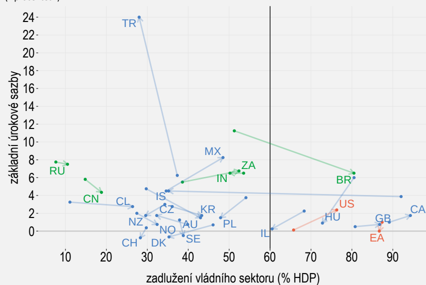
Graf 5 – Změna velikosti relativního prostoru ve fiskální a monetární oblasti
